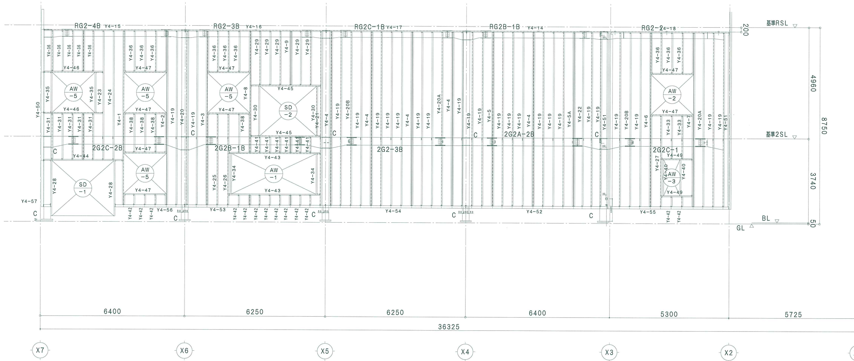
X ← Y4通り脚縁図 1/50
